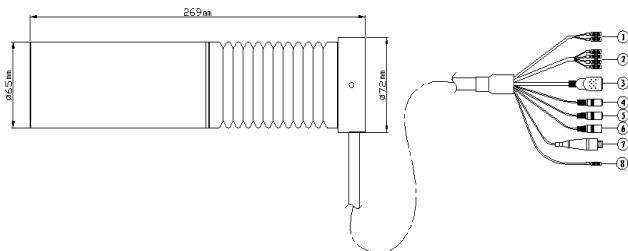
侧面图
